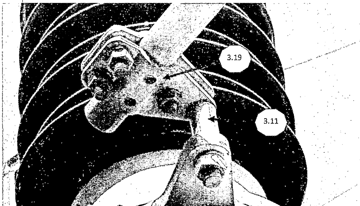
Слика бр.9: Веза моторног погона и растављача (детал повезивања управљачке спојне полуге растављача и ротационог диска женске руке)
