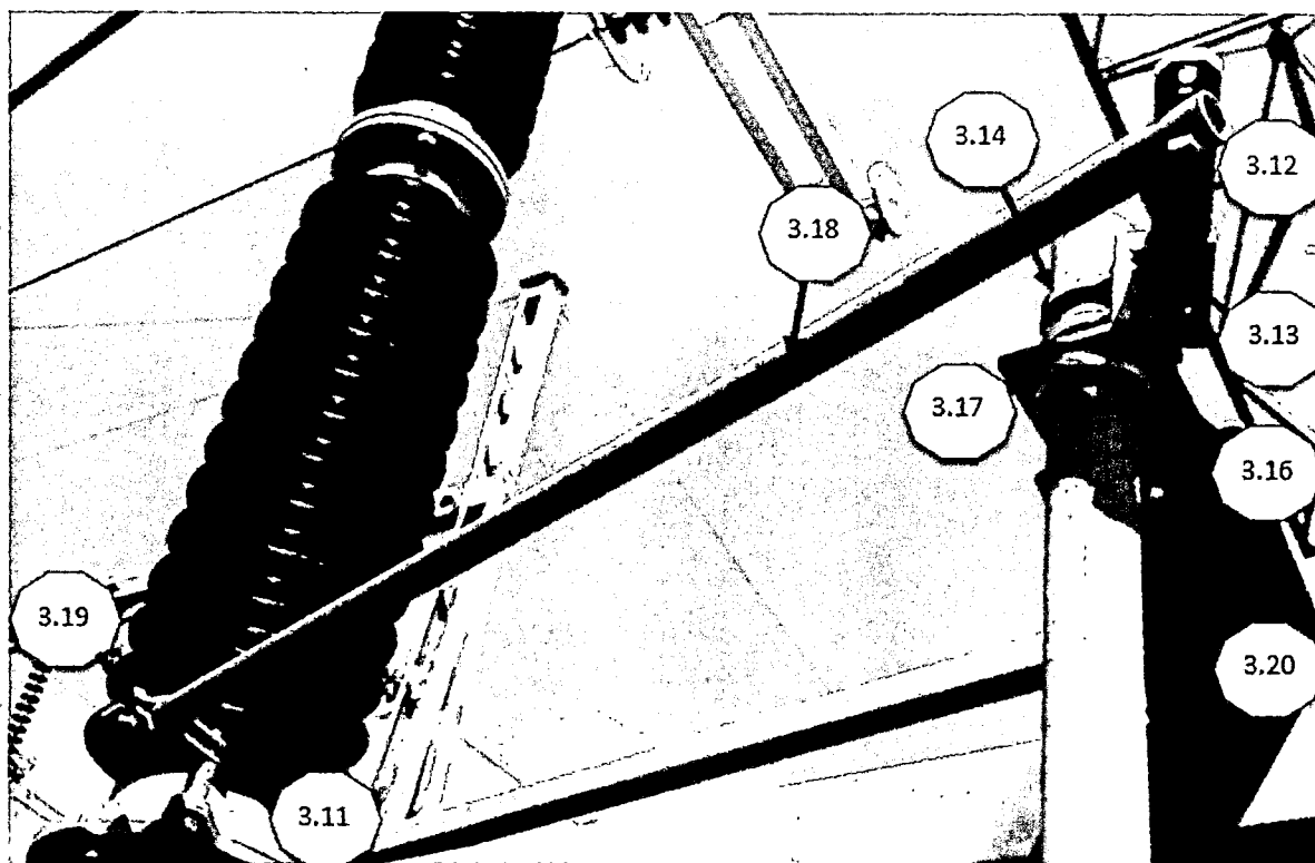
Слика бр.7: Веза моторног погона и растављача Picture 7: Connection between motor drive and disconnect mechanism
