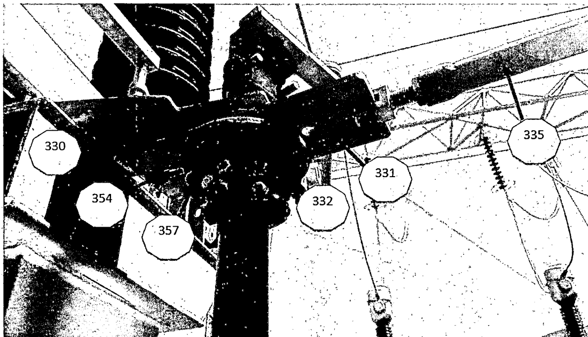
Слика бр.11: Механичка међублокада између два моторна погона (деталј монтаже блокаде на излазно вратило моторног погона)
