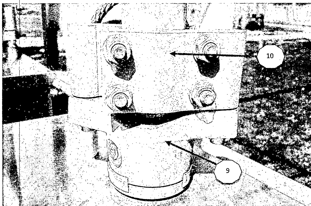
Слика бр.10: Веза моторног погона и растављача (детал повезивања вратила моторног погона и излазног вратила – преко носача спојне клеме _поз.9, и спојне клеме _поз.10)
