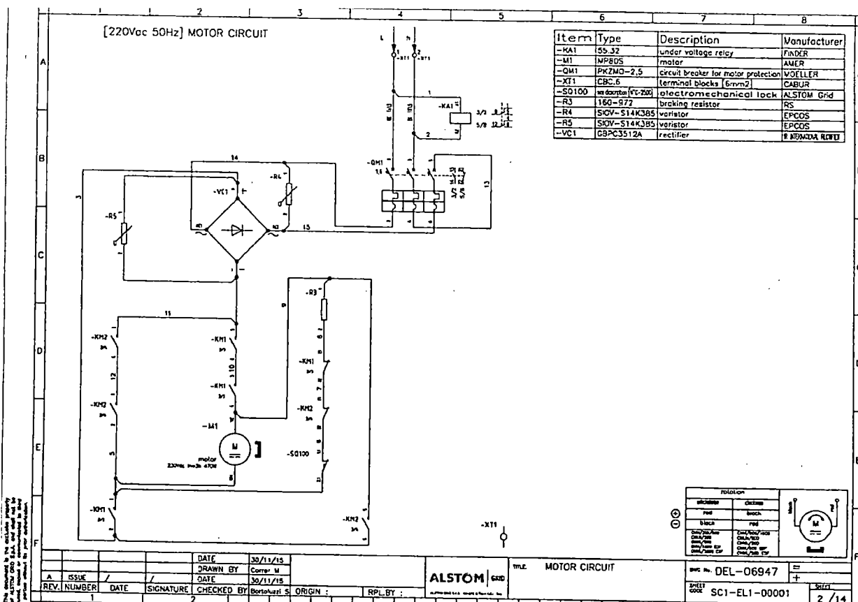
Слика бр.4: Напајање мотора растављача 220VAC 50Hz (Исечак из фабричке шеме DEL-06947) Picture 4: Motor circuit, 220VAC 50Hz supply (extract from original factory drawing DEL-06947)
