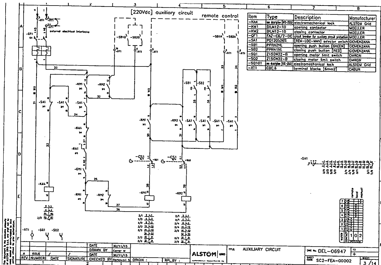
Слика бр.5: Управљачко коло растављача 220VDC (Исечак из фабричке шеме DEL-06947) Picture 5: Auxiliary (control) circuit 220VDC (extract from original factory drawing DEL-06947)
