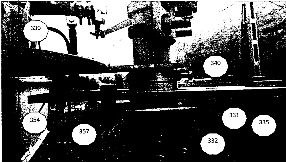
Слика бр.12: Механичка међублокада_између два моторна погона (деталъ фиксирања контролне плоче за блокаду на излазно вратило моторног погона)
